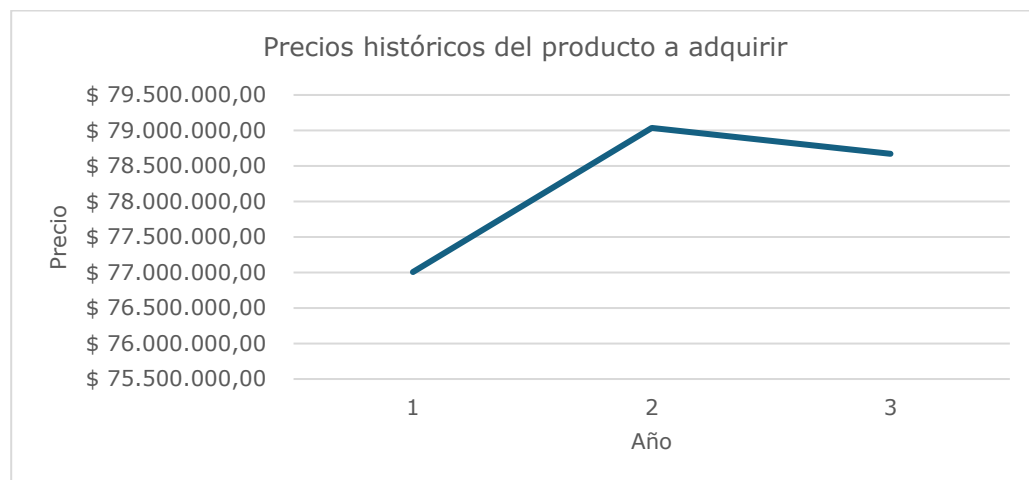
Gráfica 2. Ejemplo de gráfico de línea.
