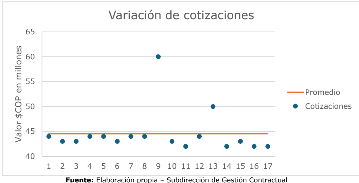
Gráfica 7. Comparación del valor de las cotizaciones con su promedio
