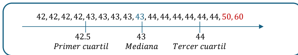
Gráfica 10. Representación de los cuartiles
