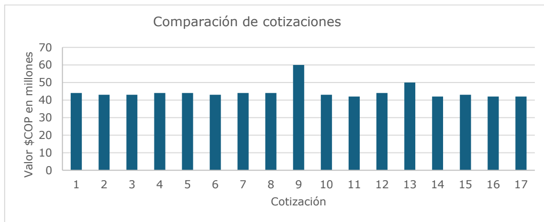
Gráfica 3. Comparación del valor de las cotizaciones con barras
