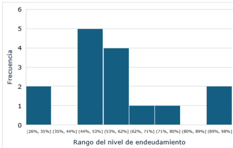
Gráfica 5. Histograma del nivel de endeudamiento de las empresas identificadas en el sector a analizar
