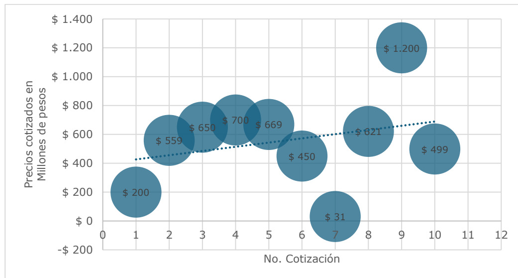
Gráfica 6. Dispersión de las cotizaciones
