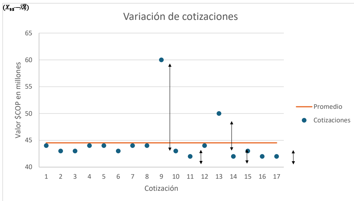
Gráfica 8. Ilustración de la distancia de los valores de cotización respecto al promedio
