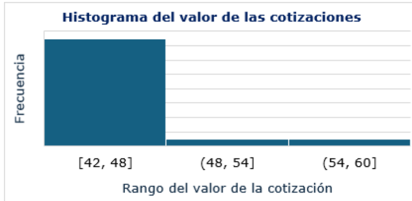
Gráfica 4. Histograma del valor de las cotizaciones
