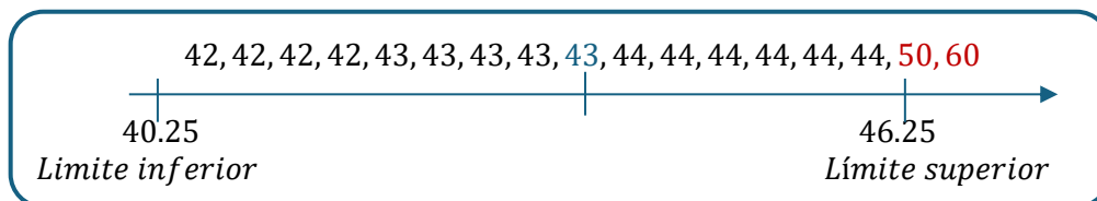
Gráfica 11. Identificación de datos atípicos
