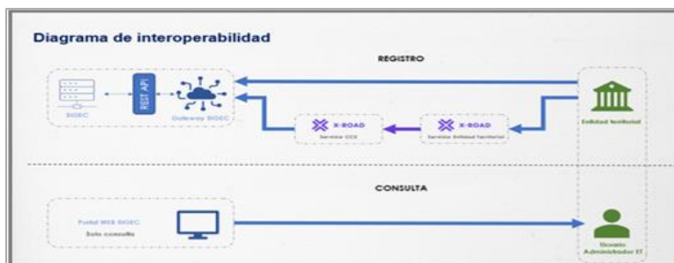
Ilustración 37: Diagrama de interoperabilidad
