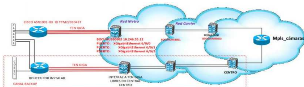
Ilustración 5. Topología de Red Final
