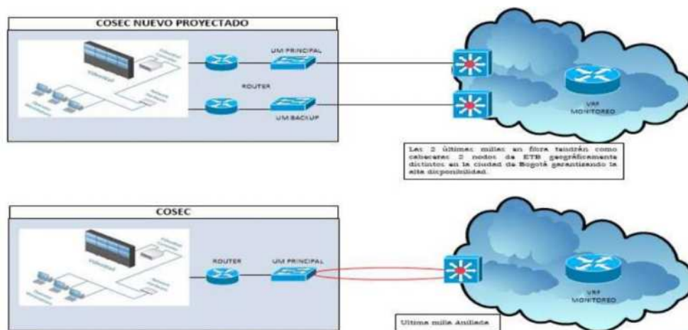
Ilustración 7. Topología De Red COSEC
